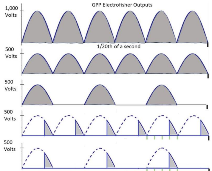
GPP エレクトロフィッシャーの出力波形
